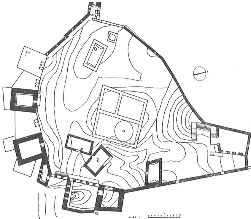
Prilog 3: Tlocrt grada Ban Vira u Trebinju 36
